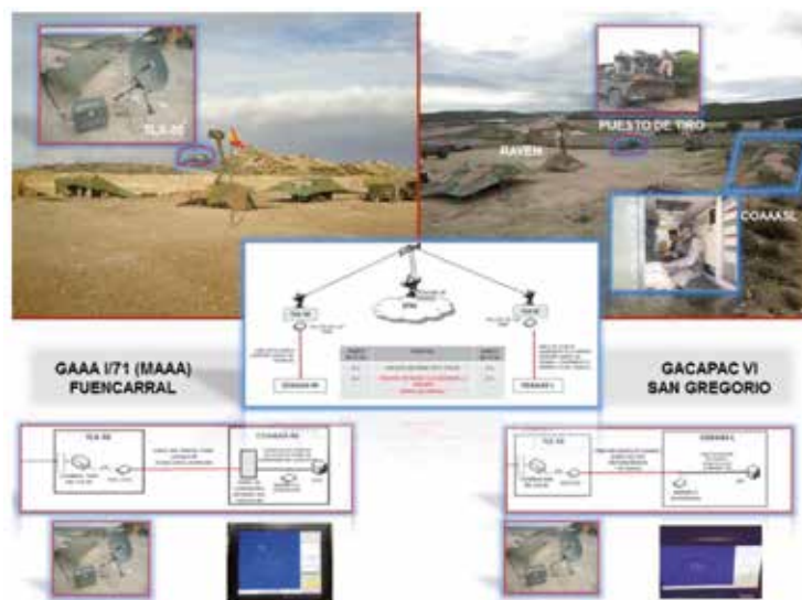
Esquema de la disposición de los medios para realizar la integración de los COAAAS Ligero y Medio mediante enlace satélite
