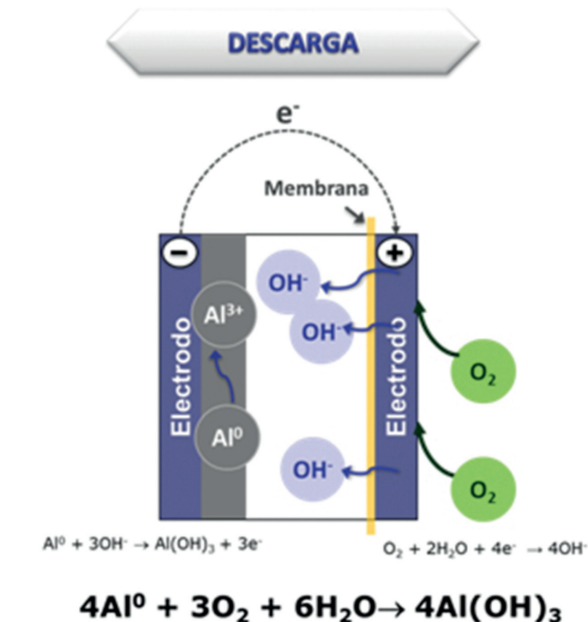
Fig. 2. Concepto de la batería aluminio-aire. (Fuente: IMDEA Energía).
