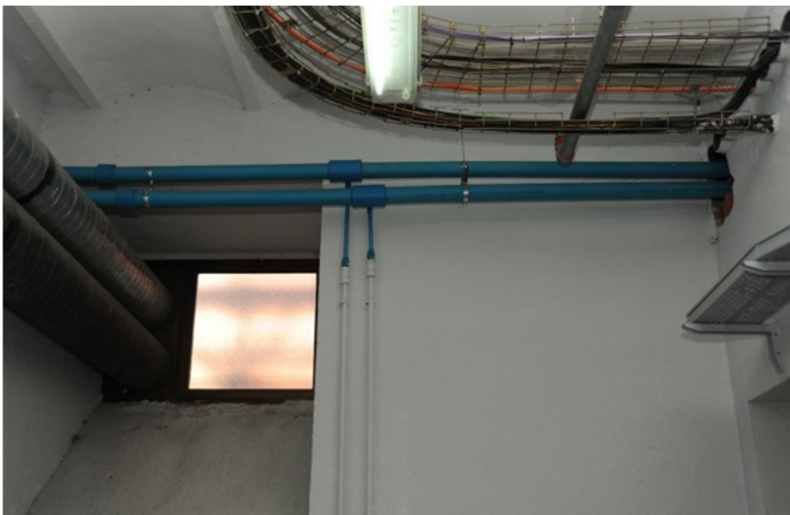
Sustitución de tuberías de calefacción de hierro por tuberías PPR y colocación de llaves de corte, en la planta sótano del edificio principal
