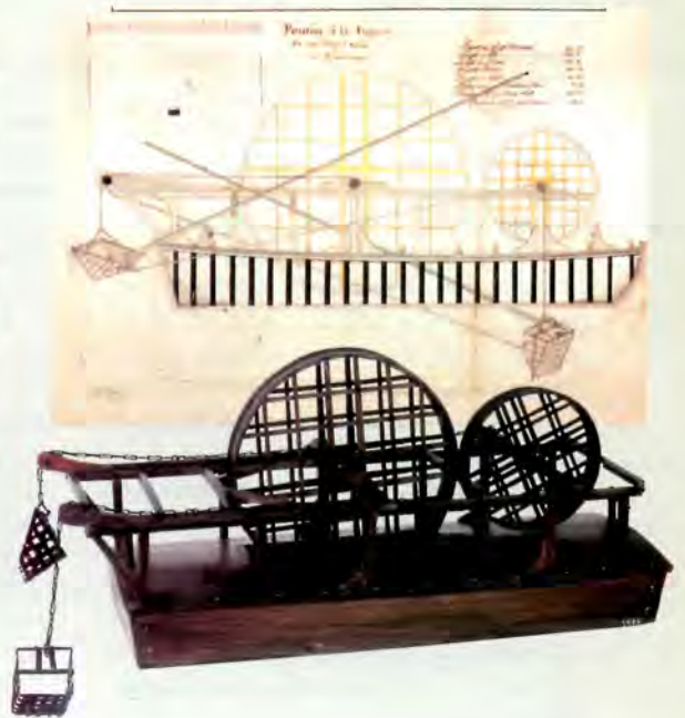
Plano de un pontón a la inglesa del XVIII para el dragado de caños y canales. Abajo, maqueta de una máquina análoga, también del XVIII.
